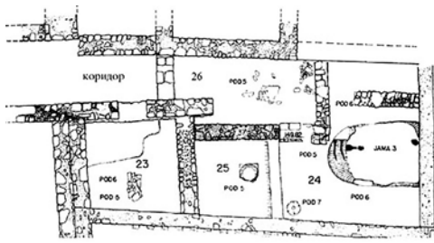
Сл.3 Домот на ГР, основа на западниот дел (според И. Микулчиќ)
