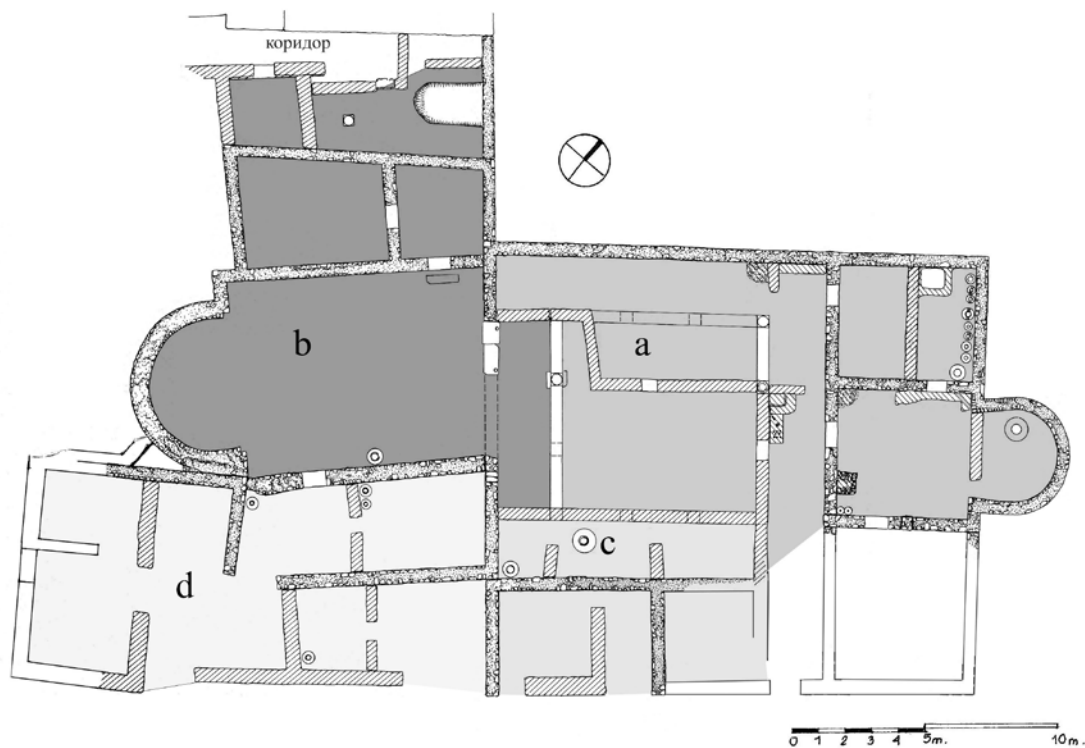
Сл.13 Основа на третата фаза од испреградениот Дом на ГР, со означени засебни станбени целини
