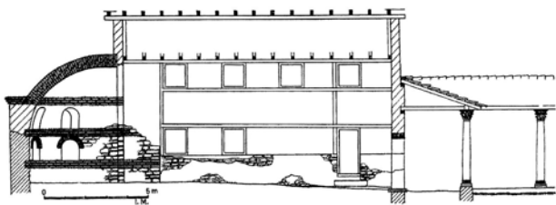
Сл.9 Домот на ГР, пресек на реконструкцијата на големата трпезарија (според И. Микулчиќ)
