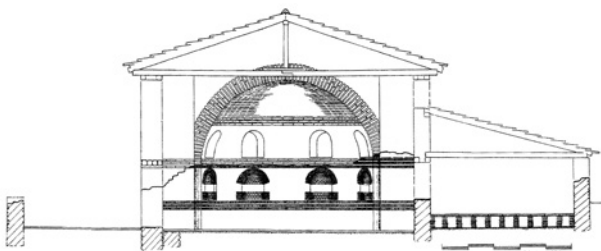
Сл.11 Пресек на југозападното крило (според И. Микулчиќ)
