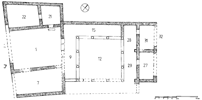
Сл.4 Домот на ГР, основа, прва фаза, доцен 3 век, (според И. Микулчиќ)
